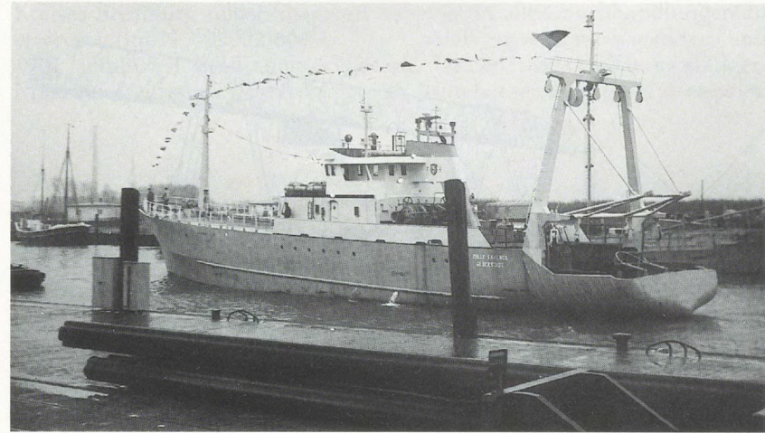
Der neue Hecklogger SG 1 „Milly Ekkenga“ läuft am 23. Dezember 1966 erstmals seinen Heimathafen Glückstadt an.
