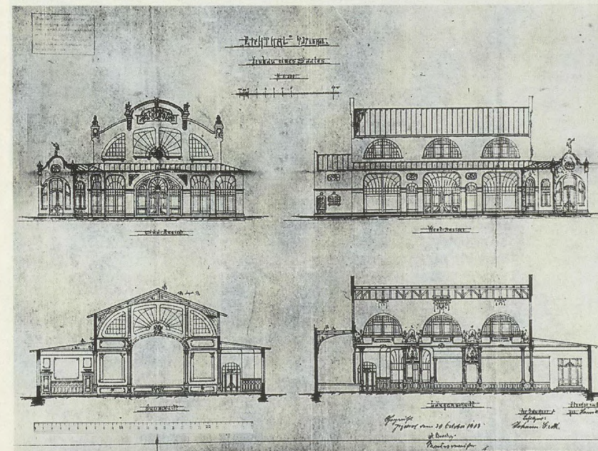
Eichthal, Architektenentwürfe 1903
