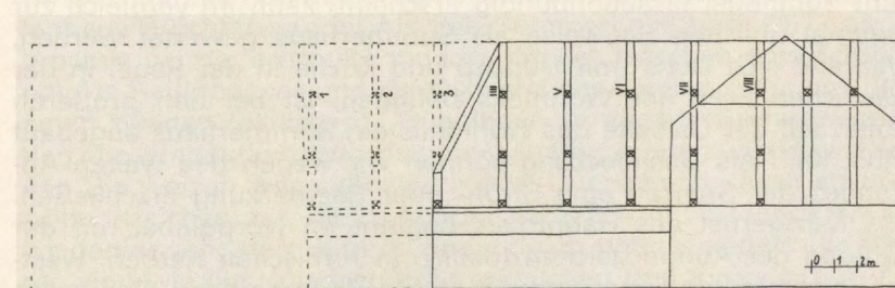
Abb. 8: Horst, Markt 9: Schemaskizze des Dachwerks, Baubestand, Längsschnitt von Westen, Kennzeichnung der Abbundzeichnung und Andeutung der Kubatur des jüngsten Flügelbaus von um 1840 (eindeutig rekonstruierbare ursprüngliche Länge des Kerngerüsts und die Größe im Jahre 1873 gestrichelt).
