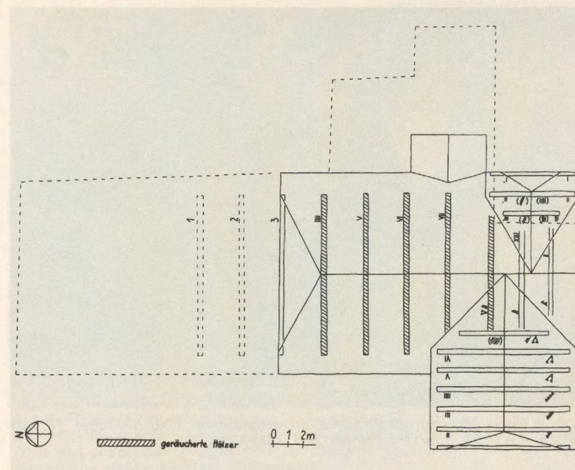
Abb. 7: Horst, Markt 9: Schemaskizze des Dachwerks, Baubestand, Grundriß, Kennzeichnung der geräucherten Hölzer und der Abbundzeichen; in Klammern diejenigen von zweitverwendeten geräucherten Hölzern, die vom ehemaligen Sommerhaus stammen (Rekonstruktion des Umrisses im Jahre 1873 gestrichelt)
