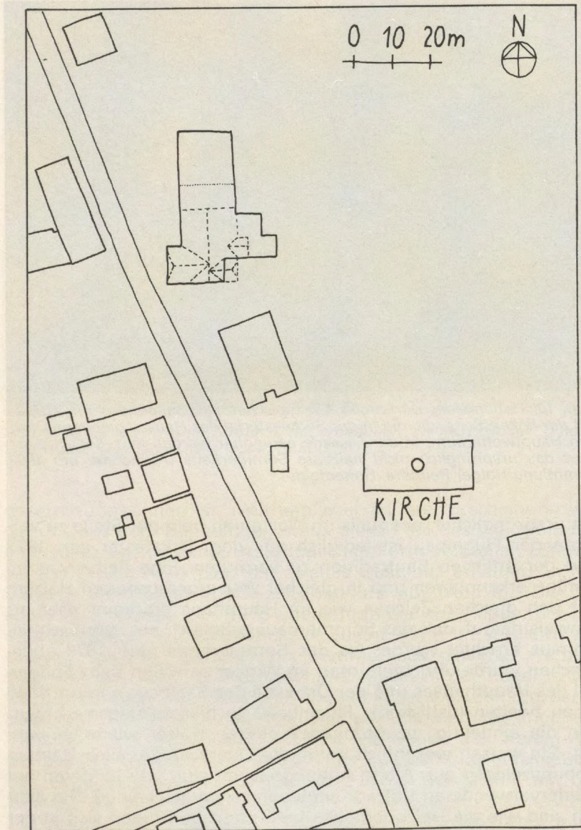
Abb. 11: Horst, Lageplan von Pienings Gasthof, um 1873, der heutige Gebäudebestand von Markt 9 ist durch gestrichelte Linien einschließlich der Firste, Grate und Kehlen hervorgehoben, die gepunktete Linie kennzeichnet die ursprüngliche Länge des bis heute erhaltenen Kerngerüsts (Umzeichnung nach der 1873 aufgenommenen Gemarkungskarte von Horst)
