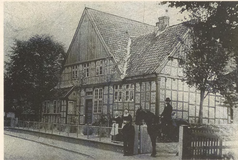
Abb. 10: Hohenfelde, Dorfstraße 65: typisches Fachhallenhaus mit Utlucht auf der linken Seite, die die in der Südwestecke des Hauses gelegene Döns, den Hauptwohnraum, in der Fassade erkennbar werden läßt, östlich angebaut das ursprünglich nicht heizbare Sommerhaus (Aufnahme um 1902, Sammlung Holger Reimers, Hohenfelde)
