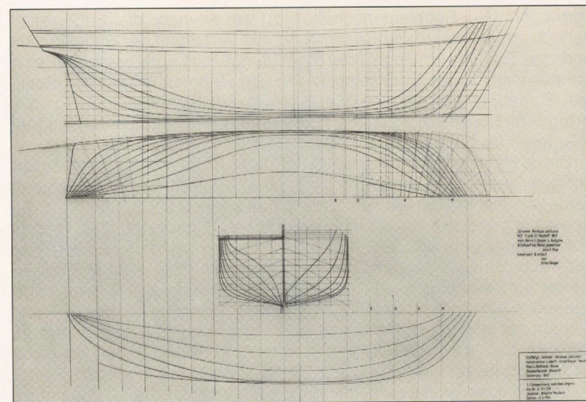
Beispiel eines Linienrisses, gezeichnet nach Entwurf von Schiffbaumeister Ernst Dreyer, Altona, für die 1847 gebauten Blankeneser Schoner „Nicolaus“ und „Lucia“. (Original im Altonaer Museum, Hamburg)
