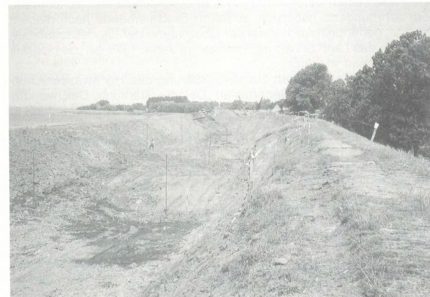
Verstärkung des Landesschutzdeiches vor Bielenberg im Jahre 1976
