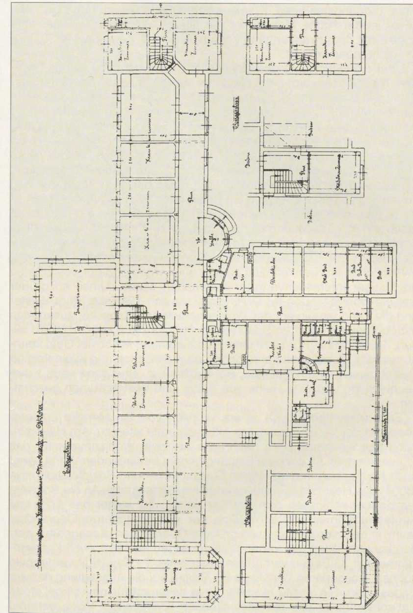
Grundriss und Raumplan des Menckestifts nach dem Neubau von 1913 (entnommen aus der Festschrift von Dr. Carlau, a.a.O.)
