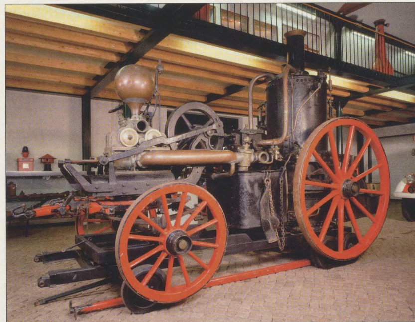
Dampfspritze „Alte Liese“ von 1869 im Feuerwehrmuseum Schleswig-Holstein, Foto: Heike Heuchert
