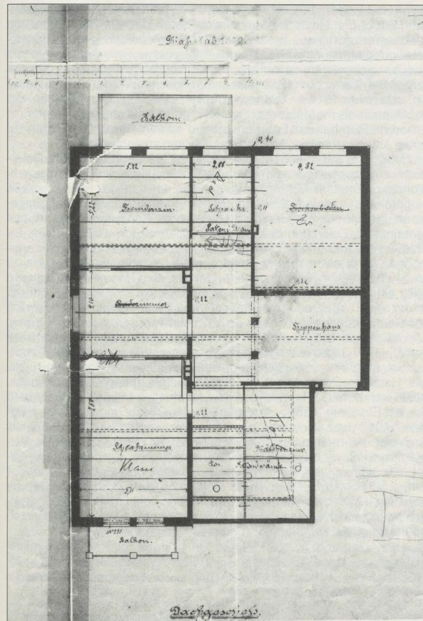
Abb. 6 Dachgeschossplan von 1899 mit ursprünglichen Raumbezeichnungen. Weitere Eintragungen wie Abb. 5.; aus dem Baugesuch (Bauaktenarchiv der Stadt Itzehoe)
