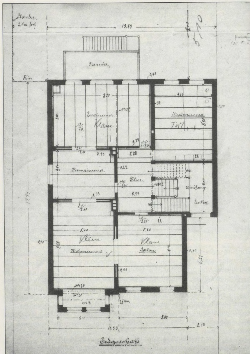
Abb. 5 Erdgeschossplan von 1899 mit den ursprünglichen Raumbezeichnungen. Spätere Eintragungen von ca. 1948 zur Umnutzung als Schule. Aus dem Baugesuch (Bauaktenarchiv der Stadt Itzehoe)
