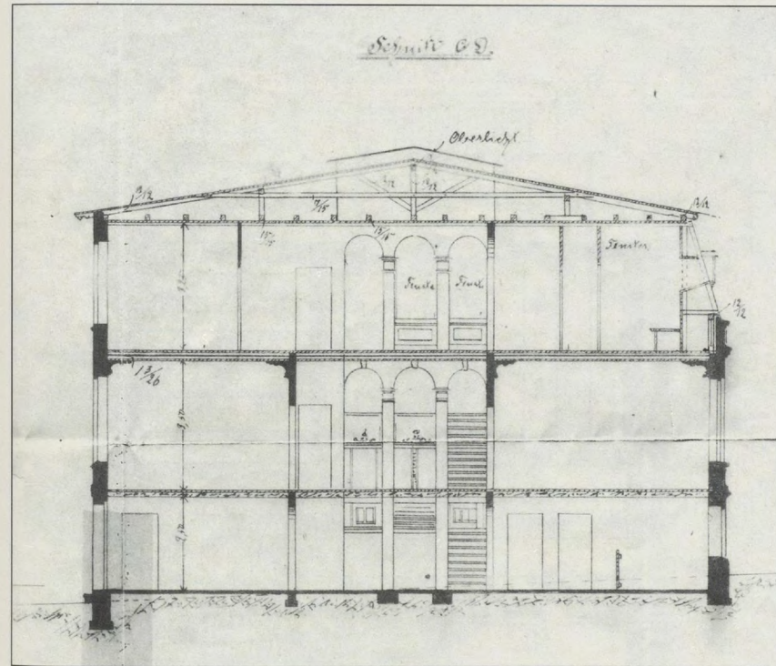
Abb. 4 Längsschnitt, rechts die Strassen-, links die Gartenseite, in der Mitte die Rundbogenarkaden des Treppenhauses, über dem rückwärtigen Gebäudeteil wurde ein Steildach ausgeführt. Aus dem Baugesuch von 1899 (Bauaktenarchiv der Stadt Itzehoe)
