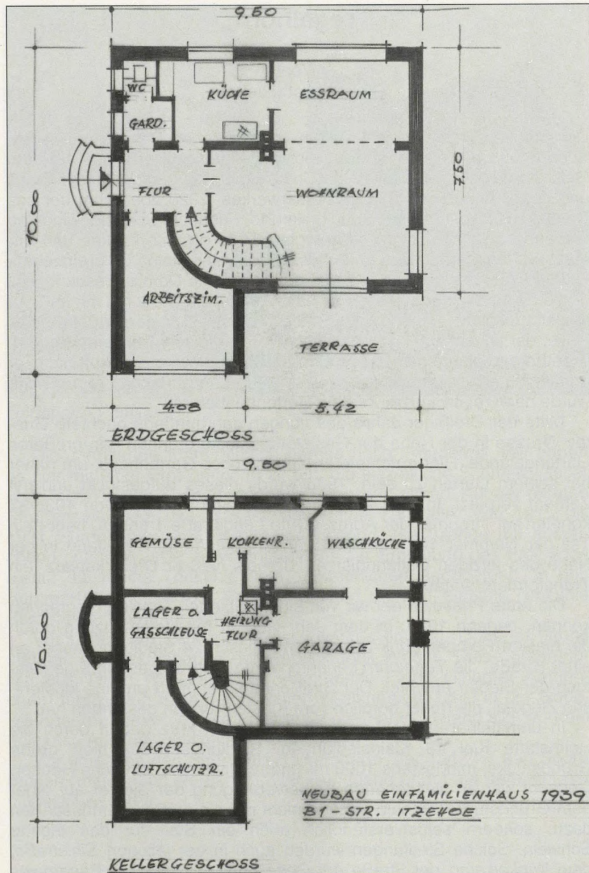
Grundriss eines Siedlungshauses 1939
