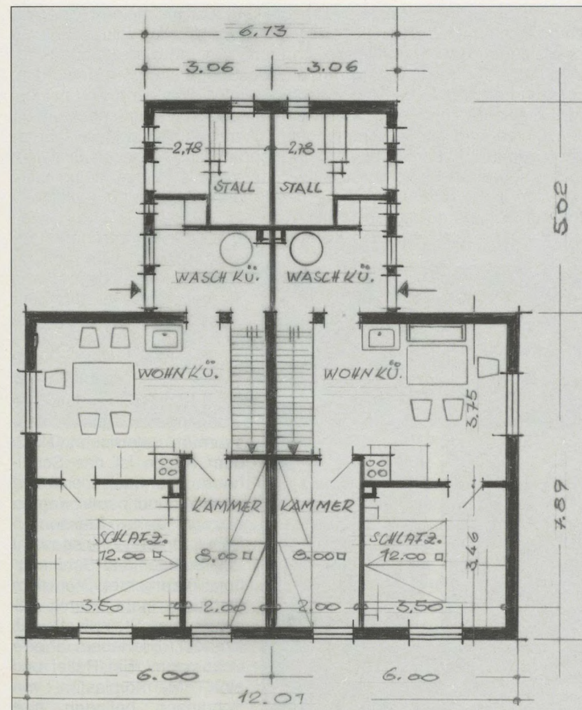
Erdgeschoss Siedlungsdoppelhaus, Kamperweg
